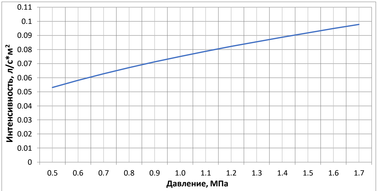
График зависимости интенсивности орошения от давления на площади 12 м 2 , защищаемой одним оросителем с высоты 2,5 м
